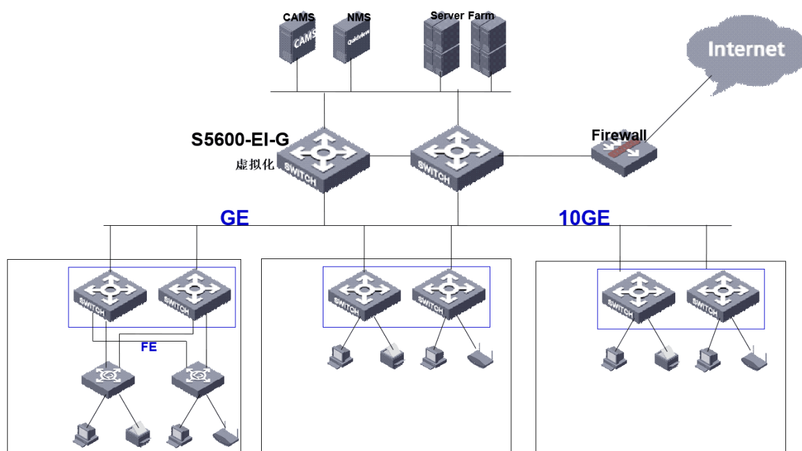
S5600-EI-G系列以太网交换机在核心层的应用
